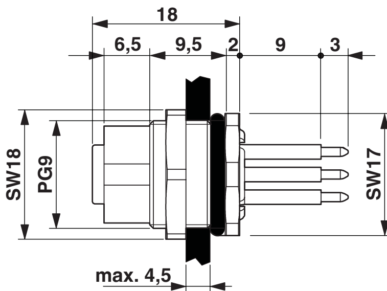
Rysunek wymiarowy
