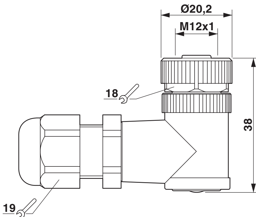
Rysunek wymiarowy
