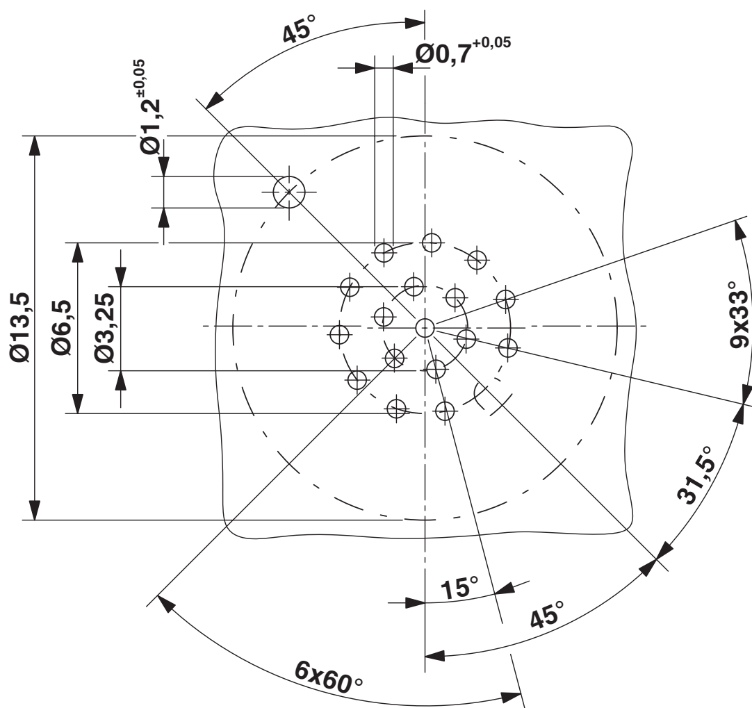
Otworowanie/geometria płytek lutowniczych
