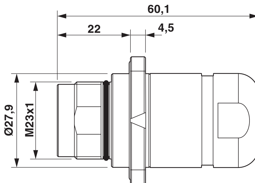
Rysunek wymiarowy
