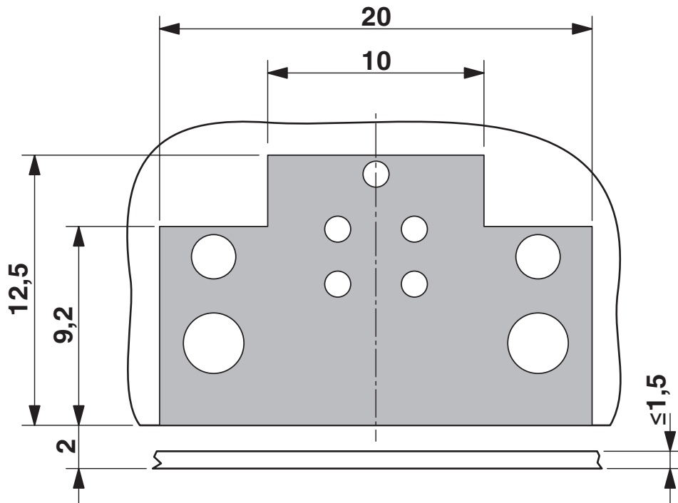
Rysunek wymiarowy
