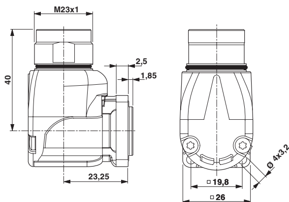
Rysunek wymiarowy
