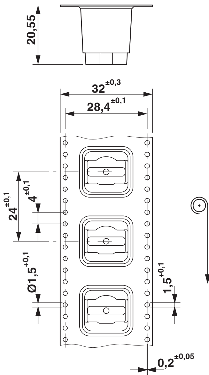
Rysunek wymiarowy
