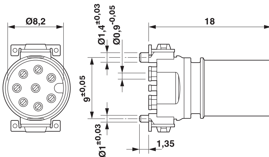
Rysunek wymiarowy
