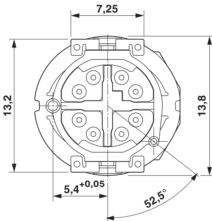
Rysunek wymiarowy
