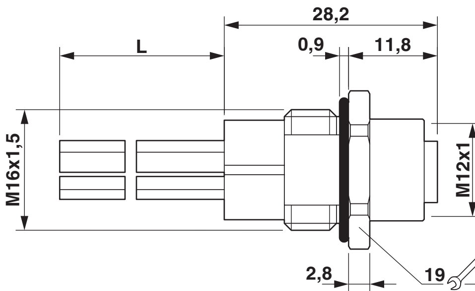
Rysunek wymiarowy
