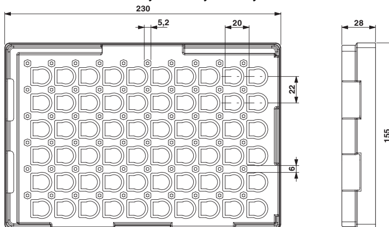
THR w przystosowanych do automatów opakowaniach Tray
