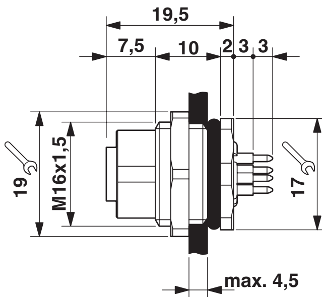
Rysunek wymiarowy
