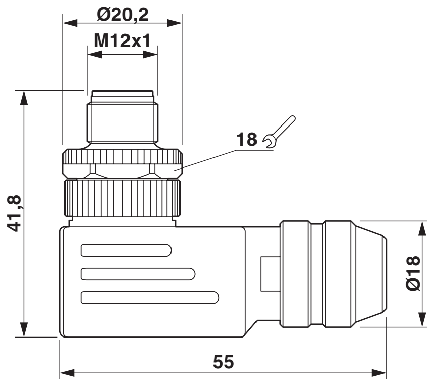
Rysunek wymiarowy
