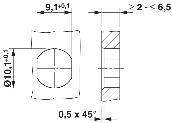
Rysunek wymiarowy
