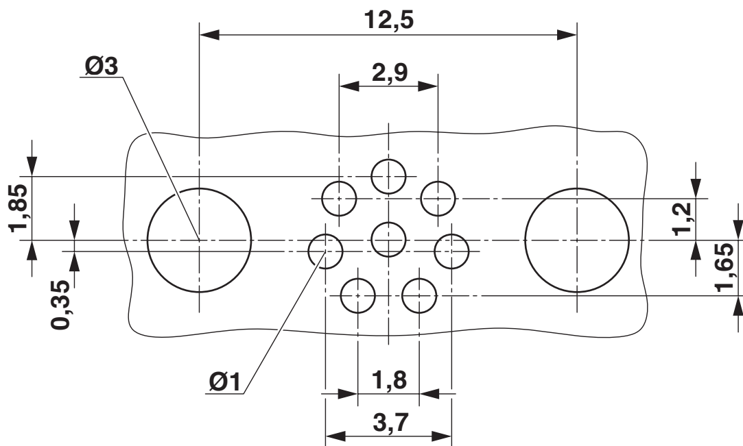
Schemat otworów w gnieździe
