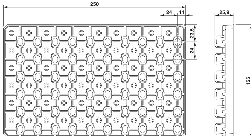
Rysunek wymiarowy
