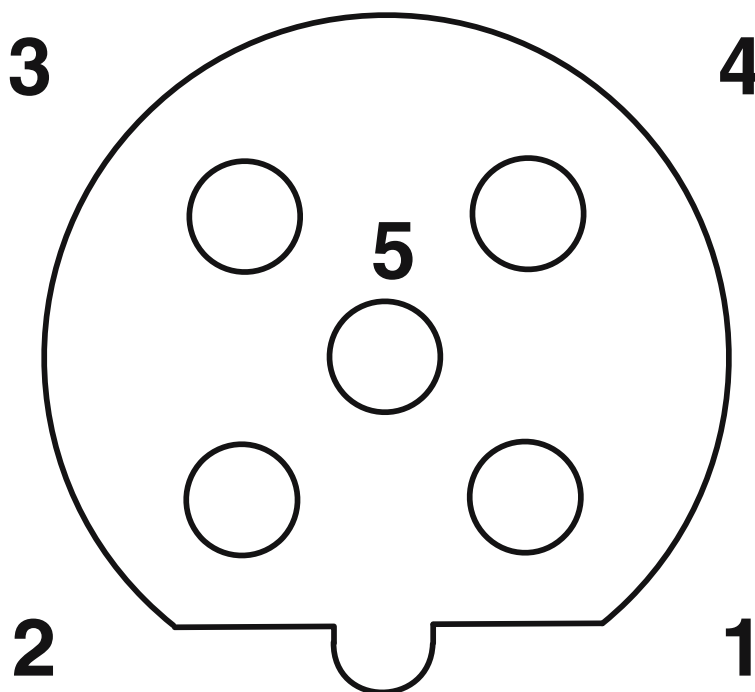
Układ biegunów wtyku z gniazdem M12, 5-biegunowy, z kodowaniem typu B, widok od strony gniazd
