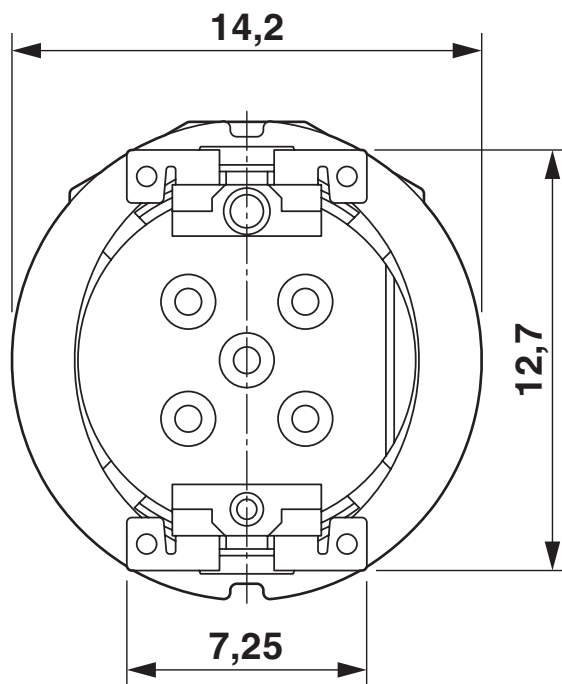
Rysunek wymiarowy
