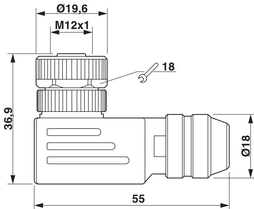
Rysunek wymiarowy
