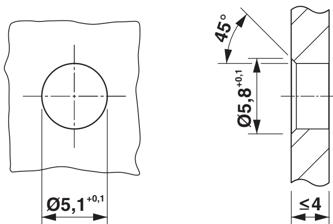
Otworowanie/geometria płytek lutowniczych
