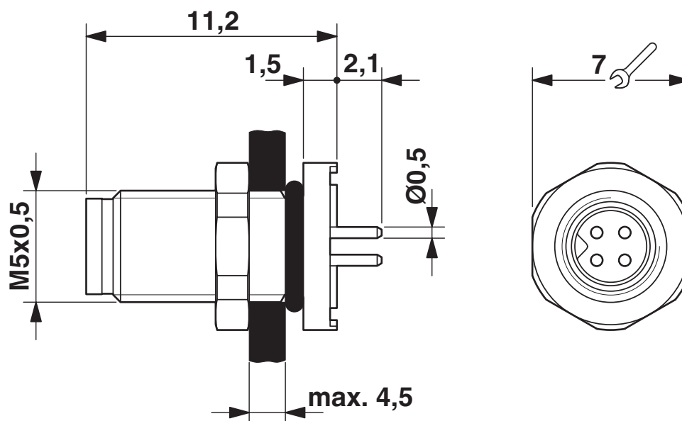
Rysunek wymiarowy
