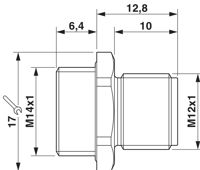
Rysunek wymiarowy
