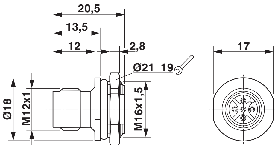
Rysunek wymiarowy
