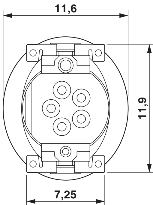
Rysunek wymiarowy
