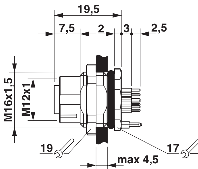
Rysunek wymiarowy
