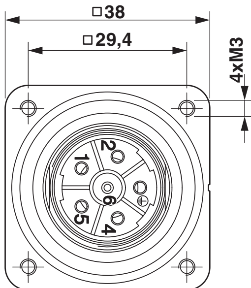
Rysunek wymiarowy
