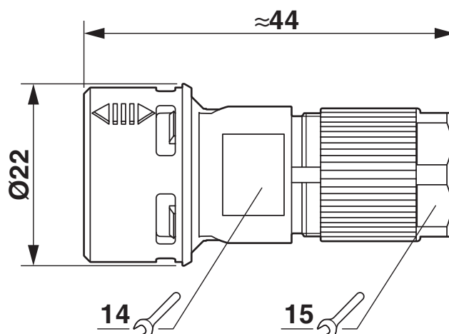
Rysunek wymiarowy
