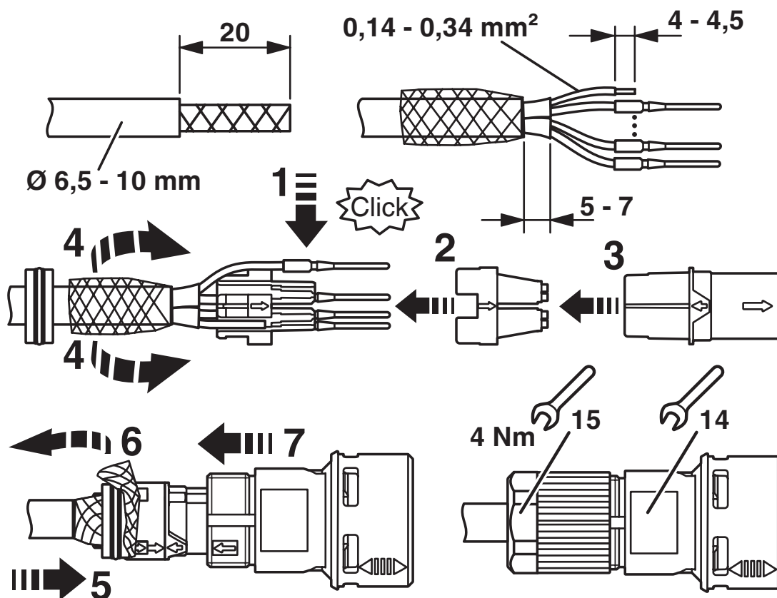
rysunek funkcyjny
