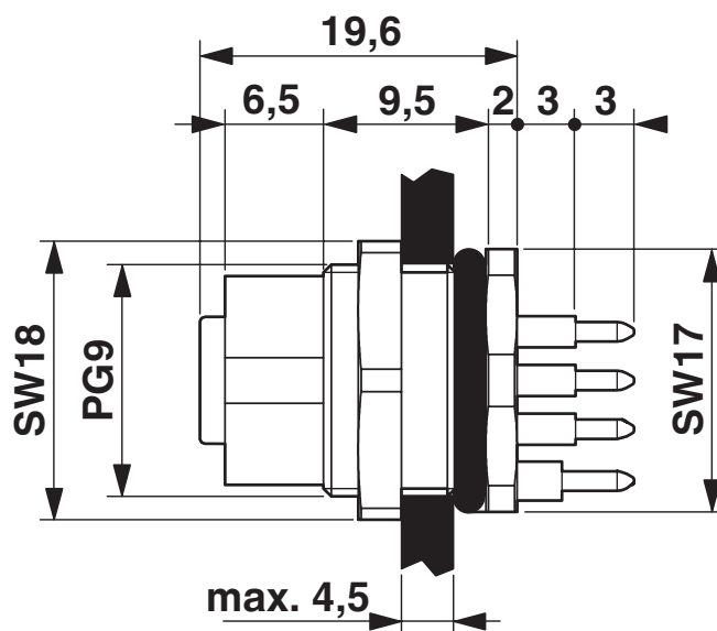
Rysunek wymiarowy
