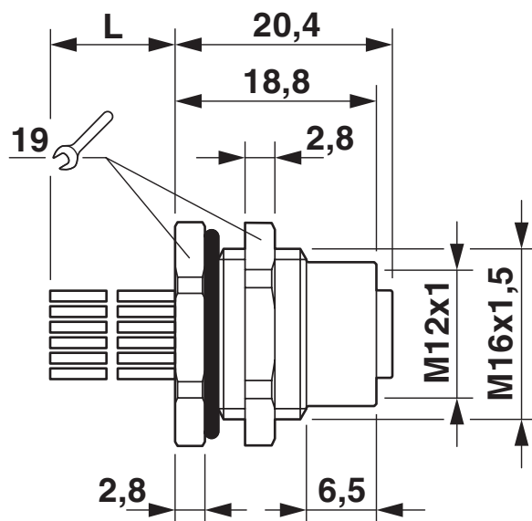
Rysunek wymiarowy
