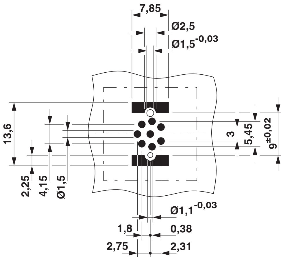
Otworowanie/geometria płytek lutowniczych
