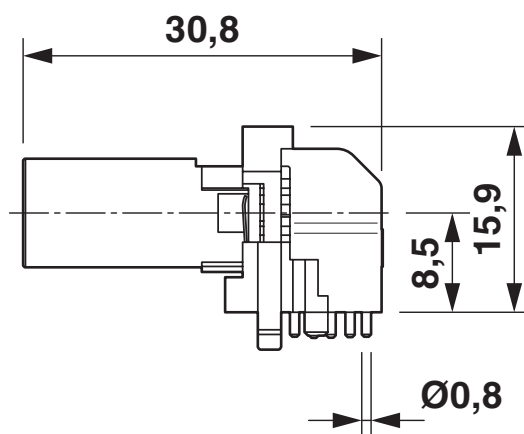
Rysunek wymiarowy
