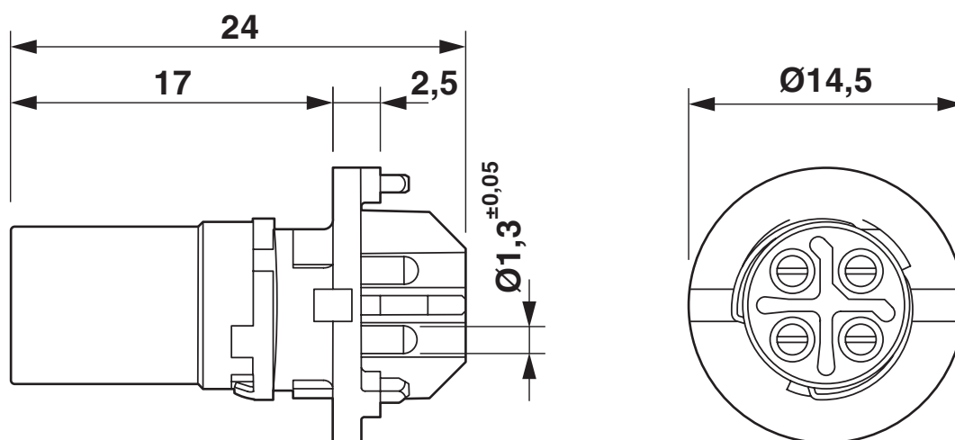
Rysunek wymiarowy
