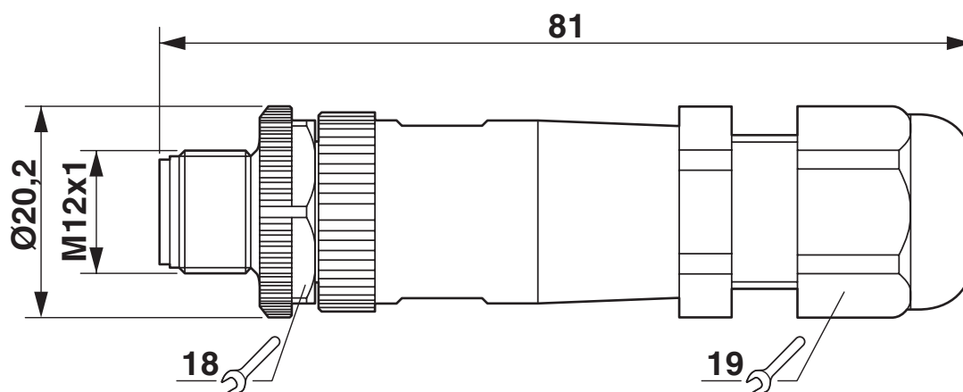
Rysunek wymiarowy
