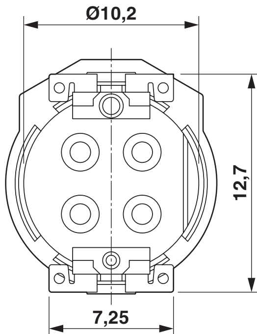
Rysunek wymiarowy
