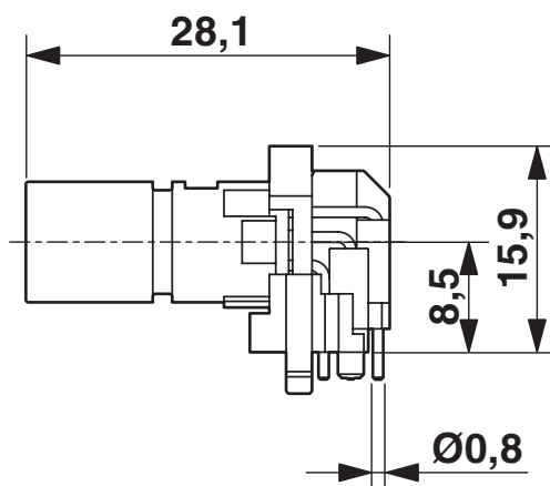
Rysunek wymiarowy
