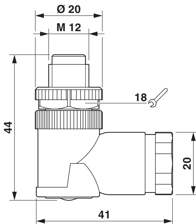
Rysunek wymiarowy
