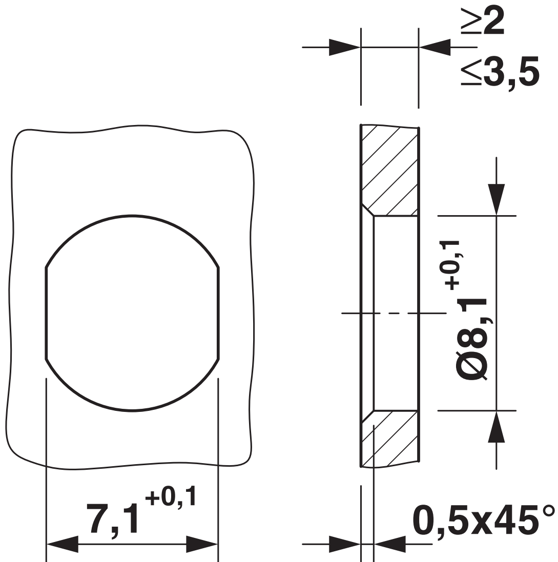
Rysunek wymiarowy
