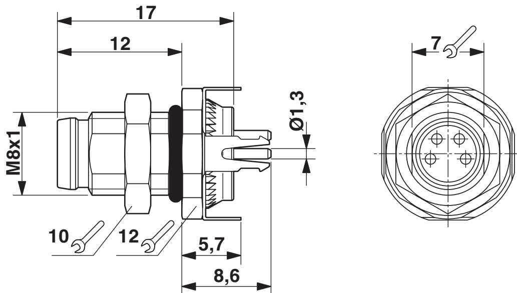
Rysunek wymiarowy
