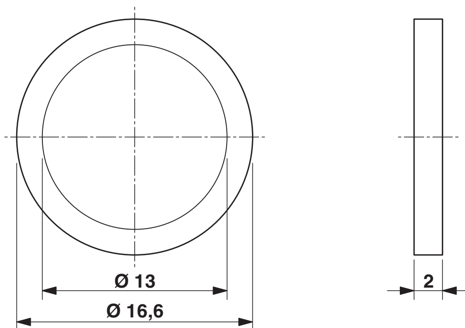
Rysunek wymiarowy
