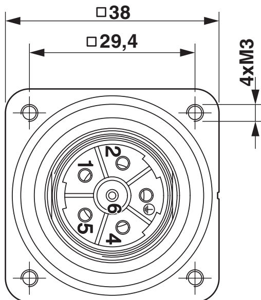
Rysunek wymiarowy
