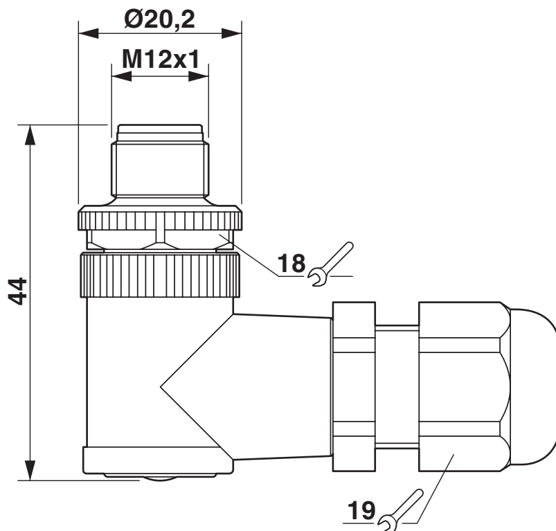
Rysunek wymiarowy
