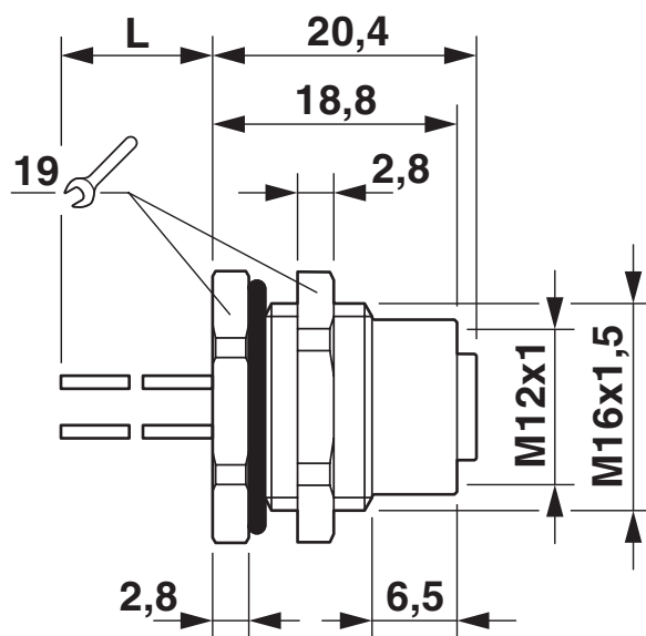
Rysunek wymiarowy
