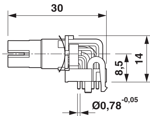
Rysunek wymiarowy
