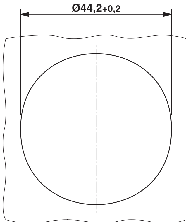
Rysunek wymiarowy
