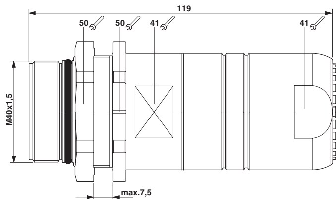
Rysunek wymiarowy
