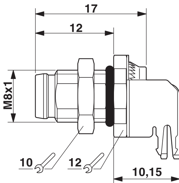
Rysunek wymiarowy
