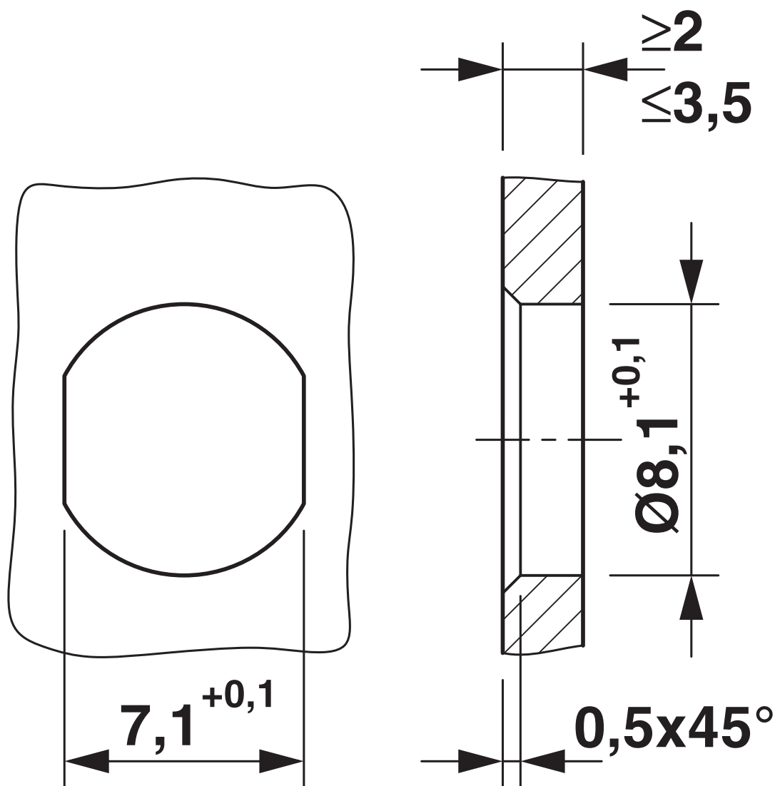
Rysunek wymiarowy
