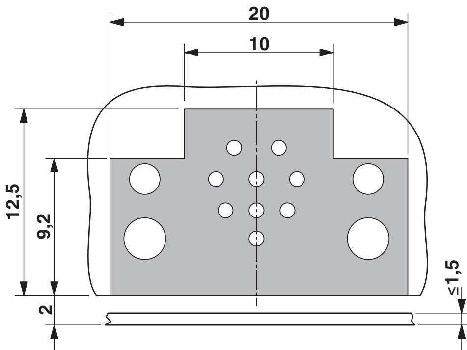
Rysunek wymiarowy
