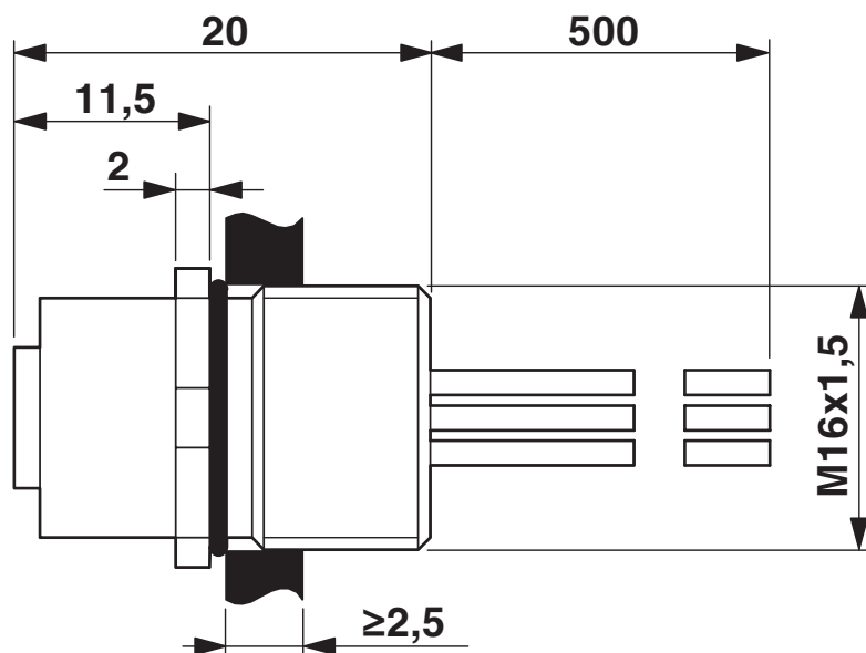
Rysunek wymiarowy
