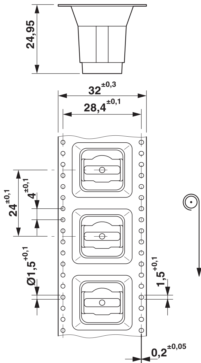
Rysunek wymiarowy
