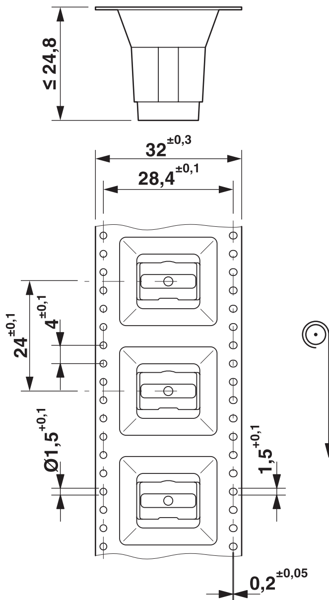
Rysunek wymiarowy
