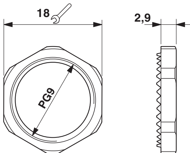
Rysunek wymiarowy
