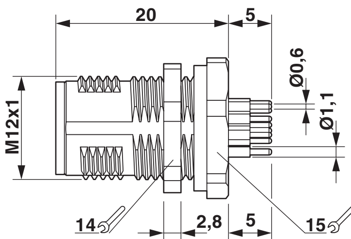
Rysunek wymiarowy
