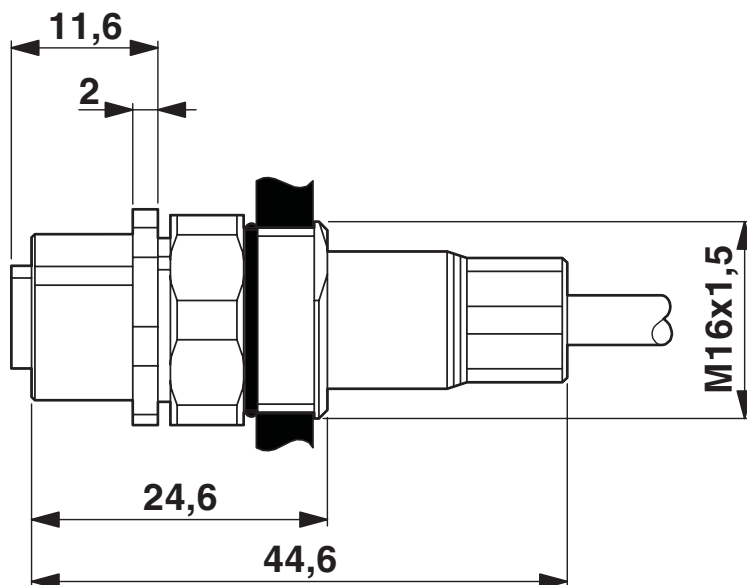
Rysunek wymiarowy
