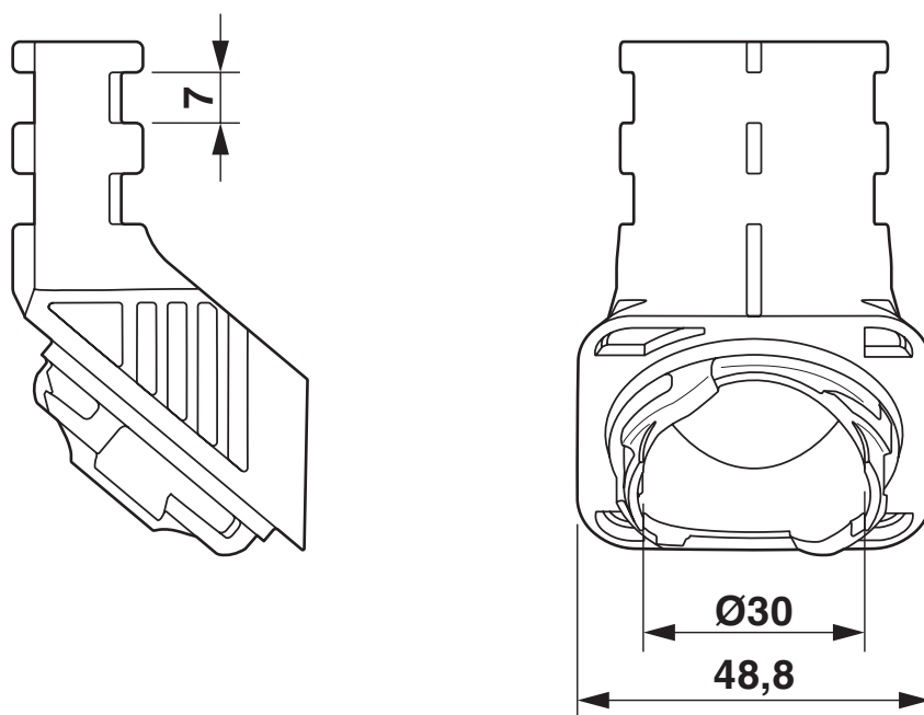
Rysunek wymiarowy
