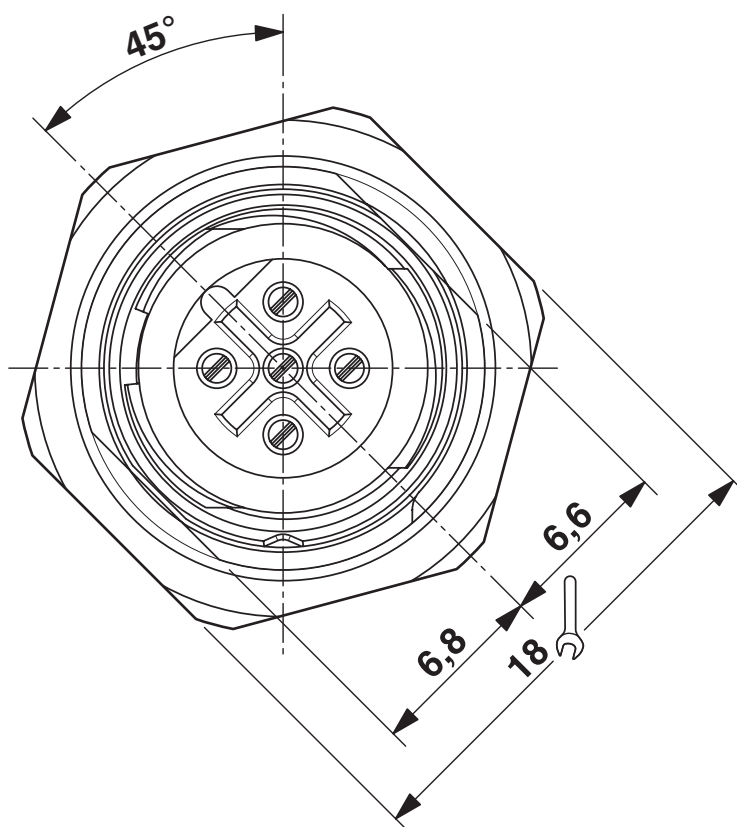
Rysunek wymiarowy
